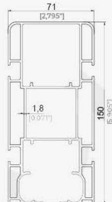
71x150 Ray Profili 71x150 Rail Profile Büküme Uygundur.
